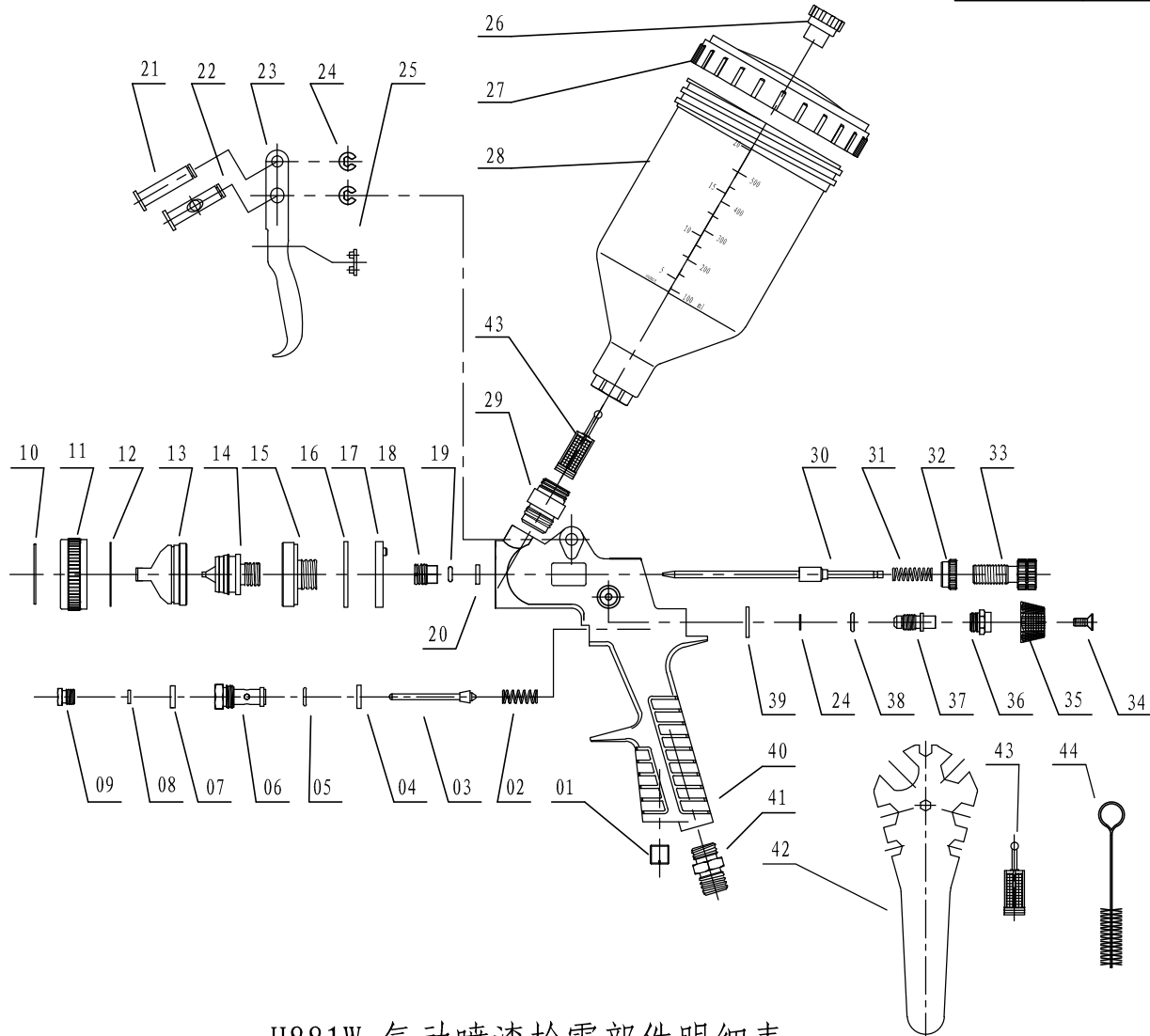
H881W 气动喷漆枪零部件明细表
